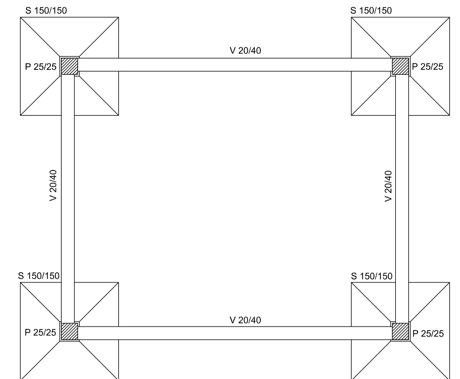
DIMENSÕES FUNDAÇÕES
