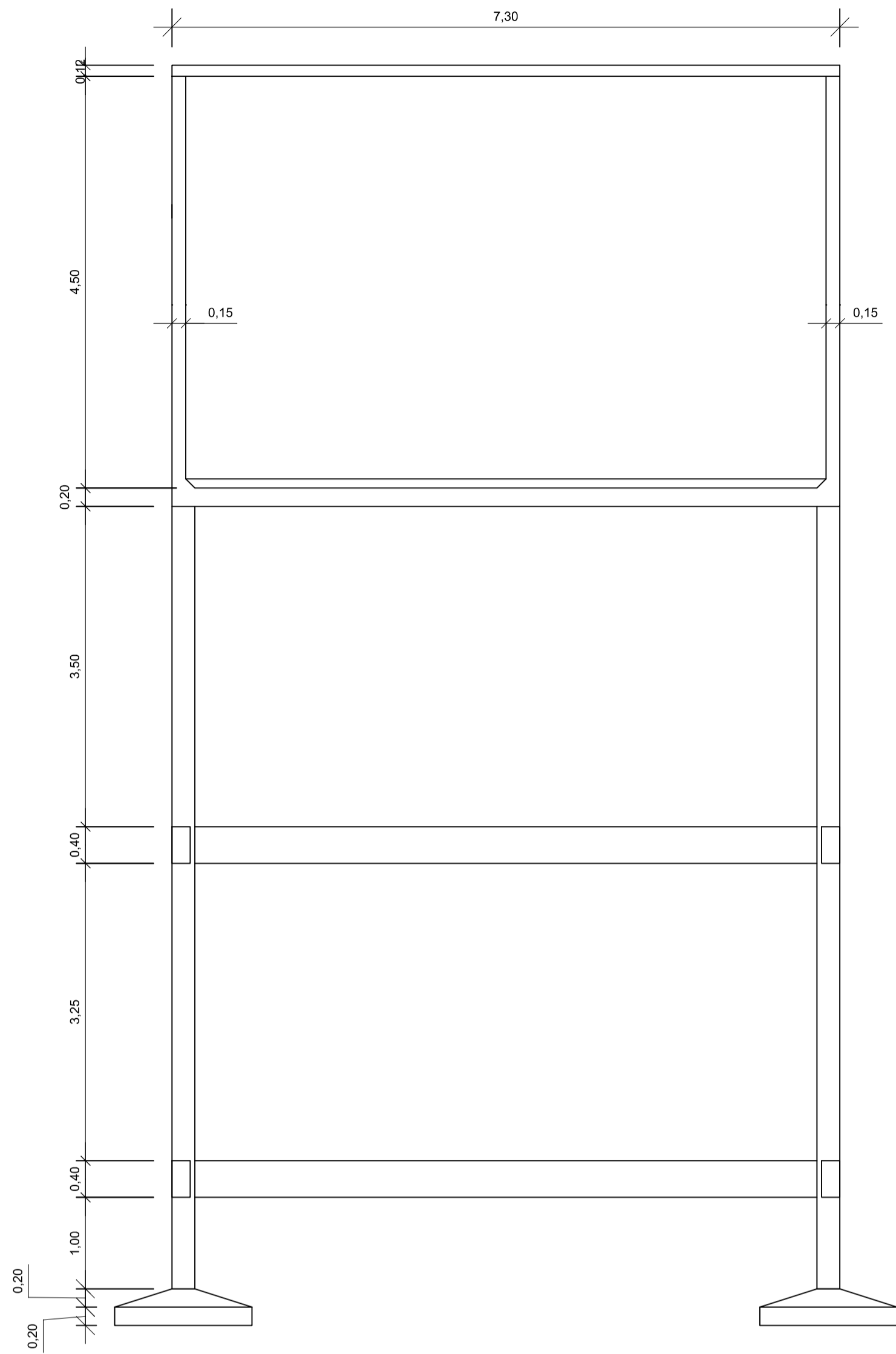
CORTE VERTICAL DO RESERVATÓRIO
