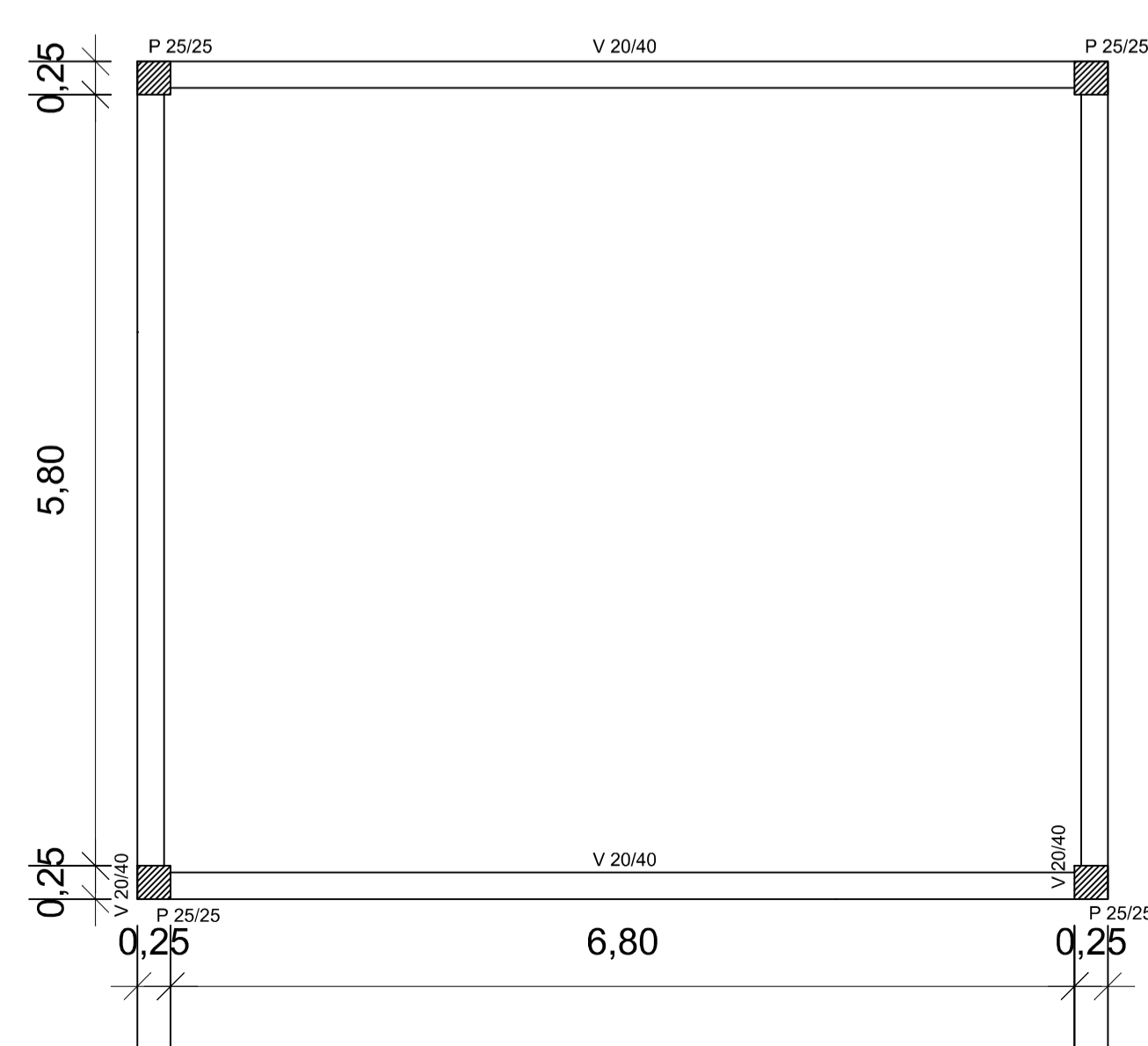
DIMENSÕES VIGAS E PILARES
